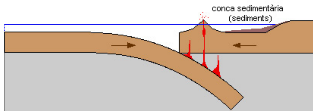
inici de la formació d'una serralada tipus andí
