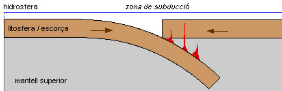
zona de subducció entre plaques oceàniques
