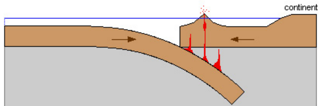
zona de subducció entre una placa oceànica i una placa oceano-continental
