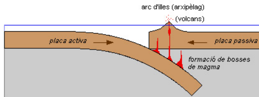
formació d'illes d'origen volcànic
