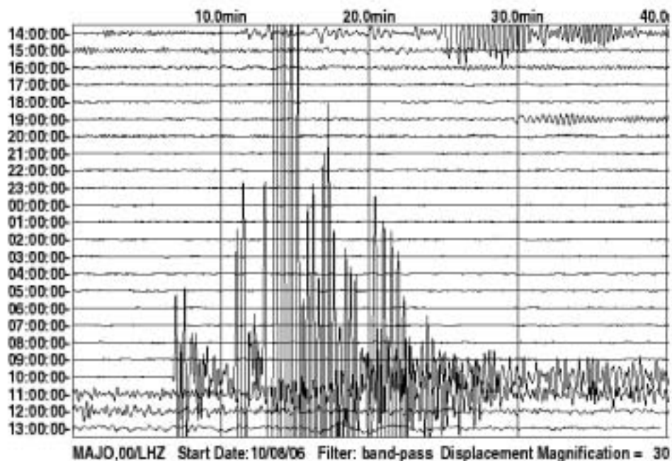
sismograma de la prova nuclear de Corea
